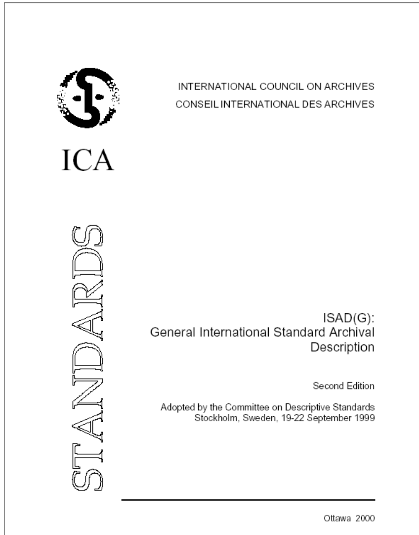
ISAD (G)
